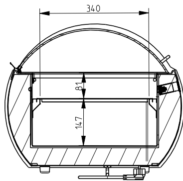
SEZIONE A-A
