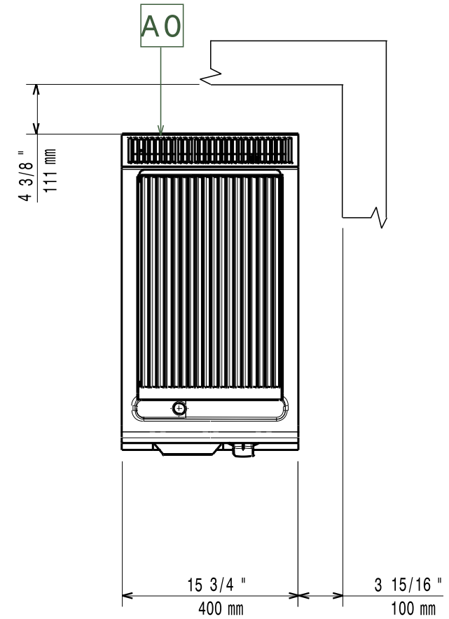
[Draufsicht]
