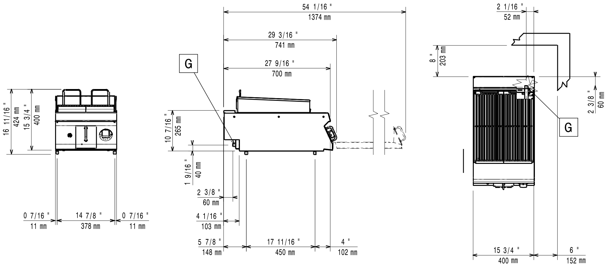
[Vorderansicht]
