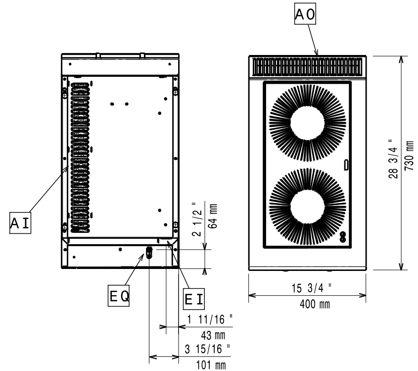
[Draufsicht]
