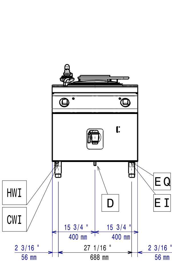
[Vorderansicht]
