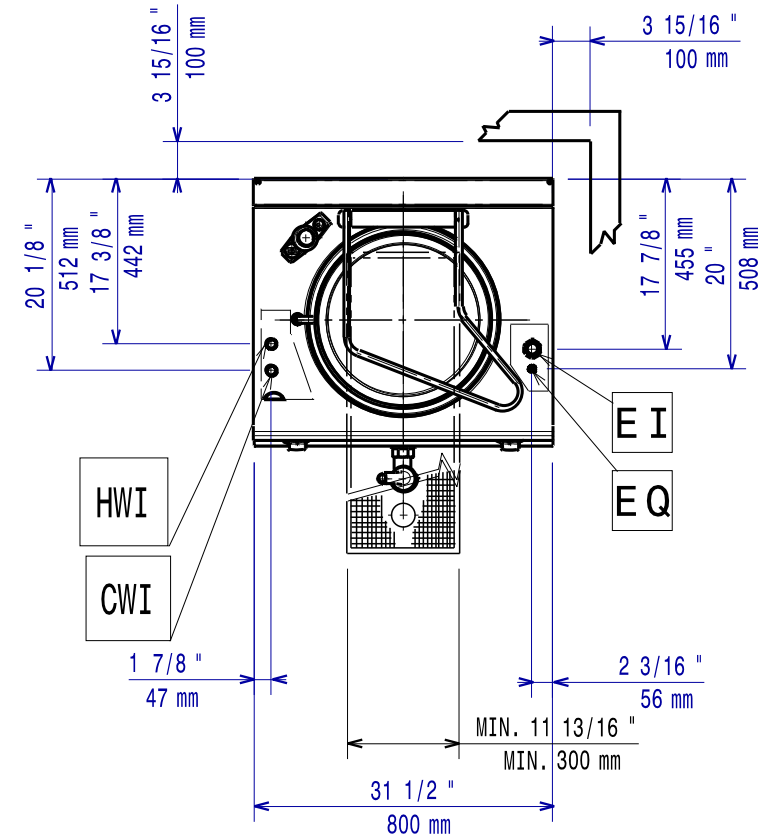
[Draufsicht]
