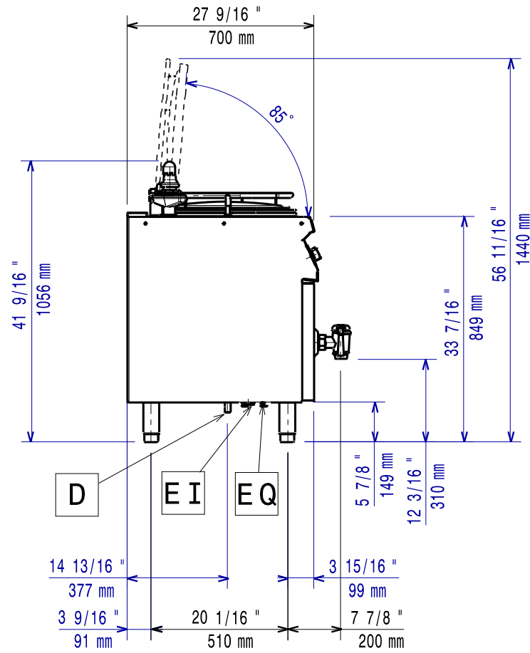
[Seitenansicht]
