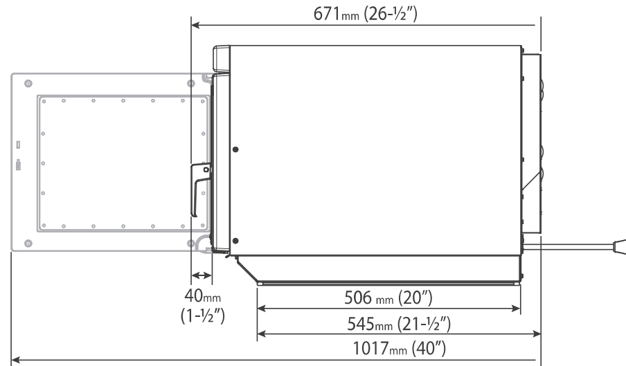
Seitenansicht
