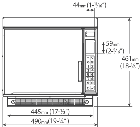
Vorderansicht
