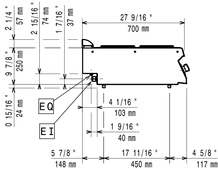
[Seitenansicht]
