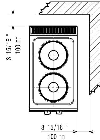
[Draufsicht]
