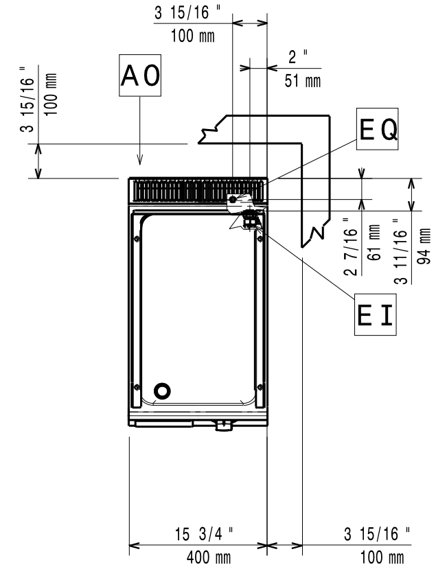
[Draufsicht]
