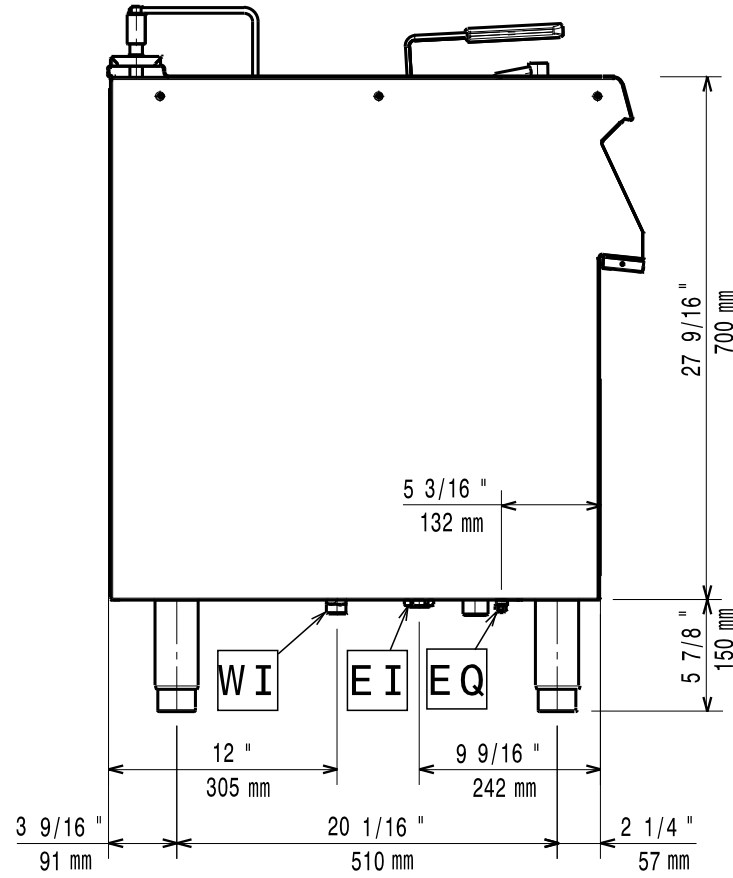
[Seitenansicht]
