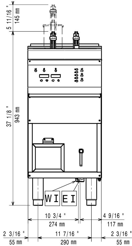
[Vorderansicht]
